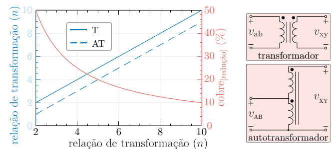
Fig. 9. Comparação da relação de ganho ( n ) do (T) e do (AT).
