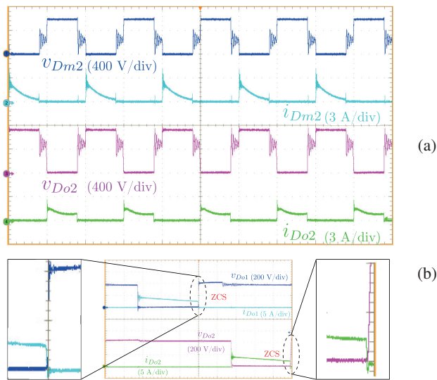
Fig. 16. Esforços de tensão nos diodos de saída, [tempo: 10 \mu s/div]. (a) Conversor II. (b) Conversor III.
