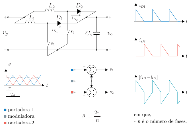
Fig. 7. Conversor boost -entrelaçado com duas fases.
