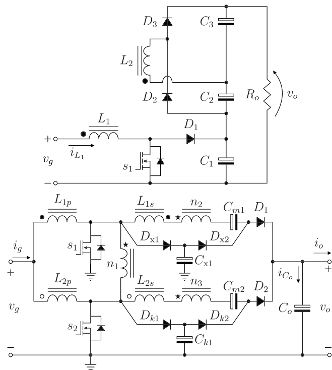
Fig. 10. Conversores com indutores acoplados e células multiplicadoras de tensão.
