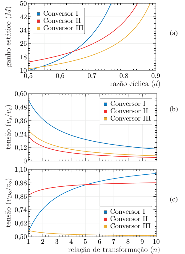
Fig. 12. Comparação de desempenho. (a) Ganho estático M_{(ccm)} . (b) Tensão normalizada ( v_s/v_o ). (c) Tensão normalizada ( v_{Do}/v_o ).
