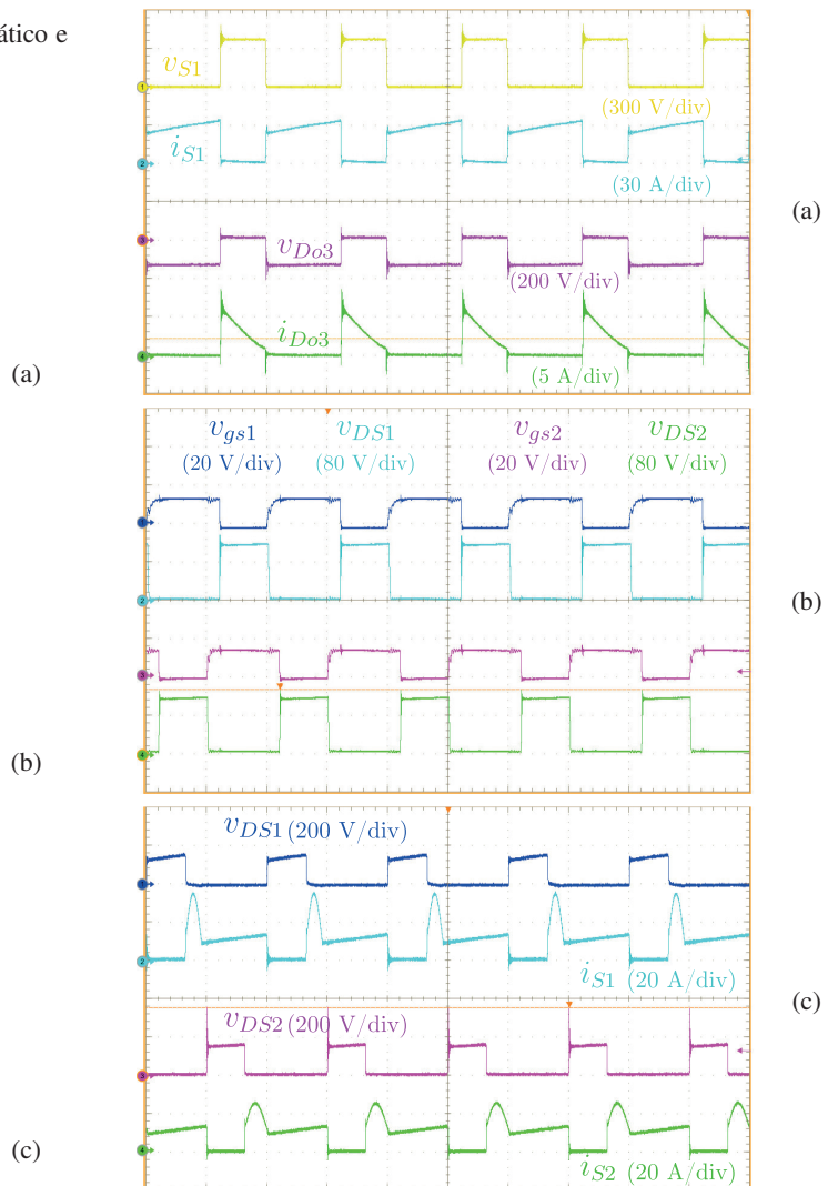
Fig. 15. Esforços de tensão e de corrente nos interruptores, [tempo: 10 \mu s/div]. (a) Conversor I. (b) Conversor II. (c) Conversor III.
