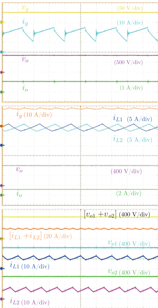
Fig. 14. Tensões e correntes: de entrada e de saída, [tempo: 10 \mu s/div]. (a) Conversor I. (b) Conversor II. (c) Conversor III.
