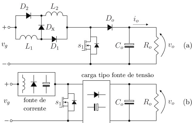
Fig. 2. Exemplo de conversores de dois estágios.
