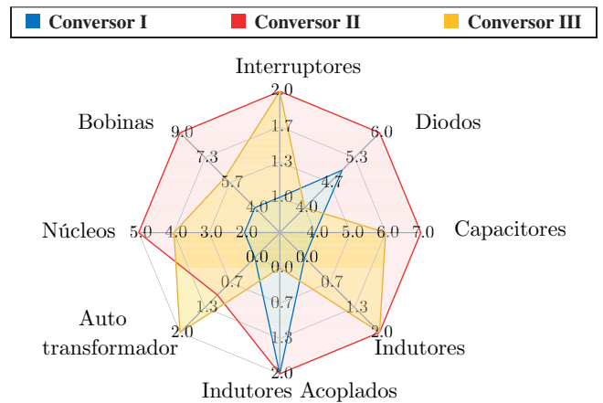
Fig. 17. Quantidade de componentes dos conversores propostos.
