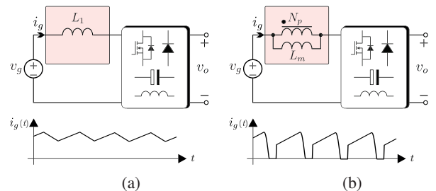
Fig. 5. Tipos de corrente de entrada para configurações monofásicas.
