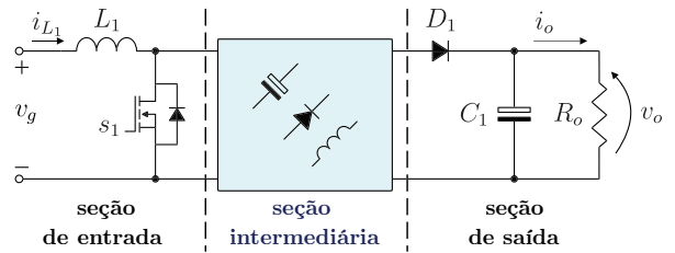
Fig. 3. Conversor com três estágios: entrada, intermediário e saída.
