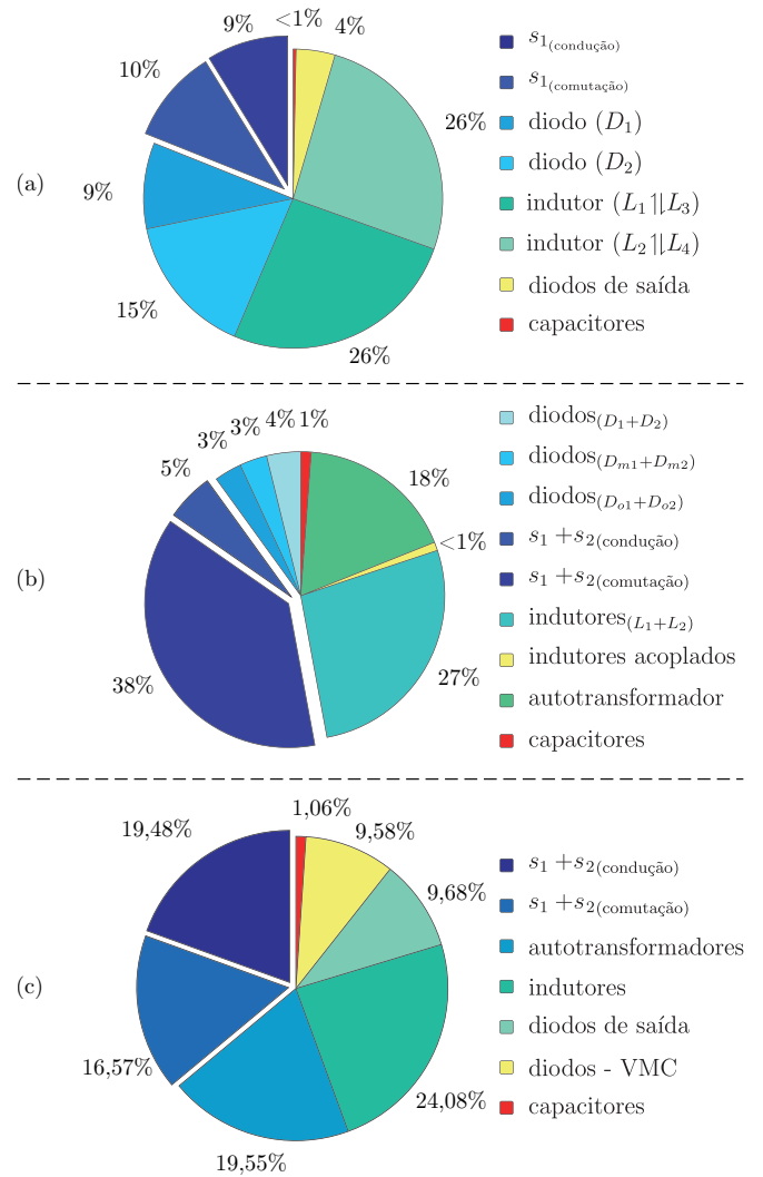
Fig. 19. Estimativa das perdas dos conversores em plena carga. (a) Conversor I. (b) Conversor II. (c) Conversor III.
