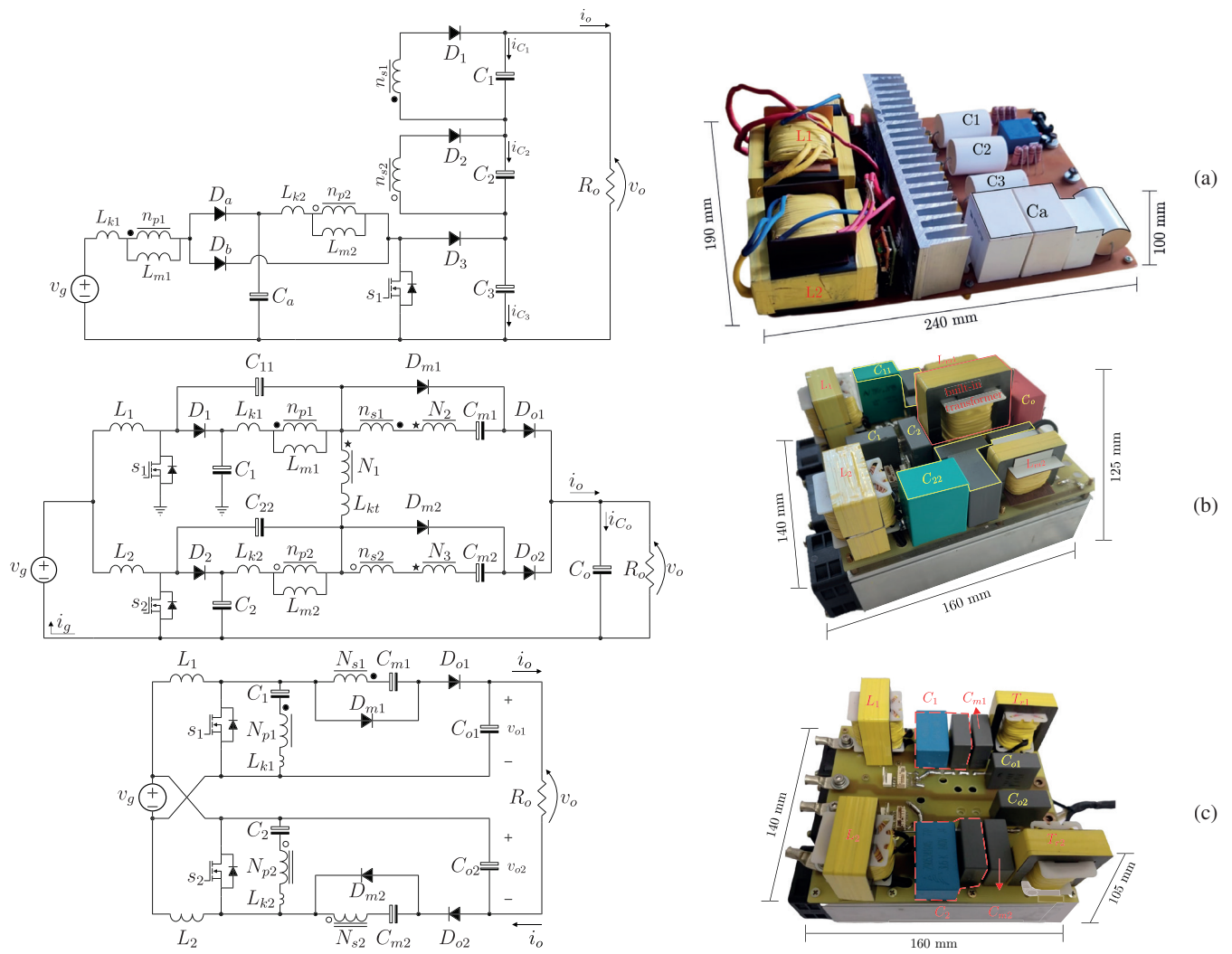
Figura 11. Circuito e fotografia dos três conversores. (a) Conversor I [14]. (b) Conversor II [15]. (c) Conversor III [16].
