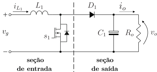
Fig. 1. Conversor com dois estágios: entrada e saída.
