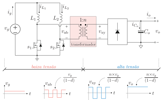
Fig. 8. Conversor boost -entrelaçado isolado.
