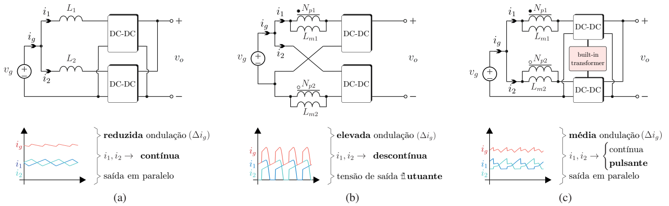
Fig. 6. Conversor boost -entrelaçado. (a) Conversor boost -entrelaçado convencional, com indutor sem acoplamento na entrada. (b) Entrada-paralela/saída-série, com indutor acoplado na entrada. (c) Entrada-paralela/saída-paralela, com indutor acoplado na entrada.
