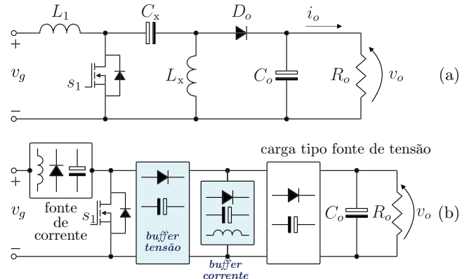
Fig. 4. Exemplo de conversores de três estágios.
