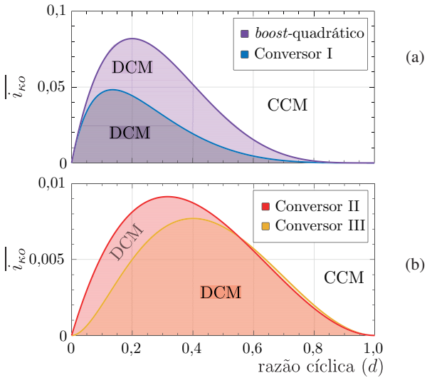
Fig. 13. Região de fronteira ( \bar{i}_{ko} ). (a) Conversor boost-quadrático e Conversor I. (b) Conversor II e Conversor III.
